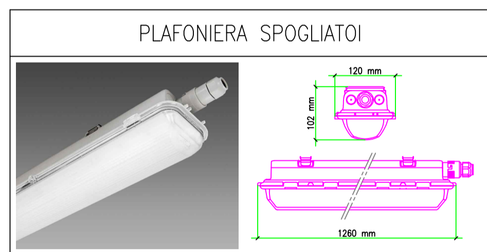
TIPICO DI COLLEGAMENTO PLAFONIERA SPOGLIATOI
