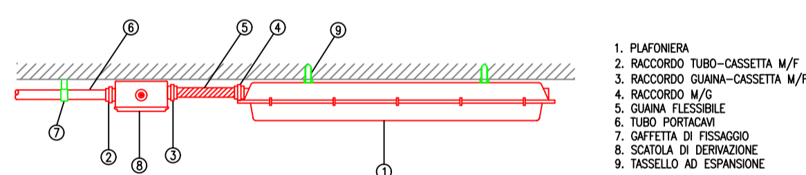
TIPICO DI COLLEGAMENTO PLAFONIERA SPOGLIATOI
