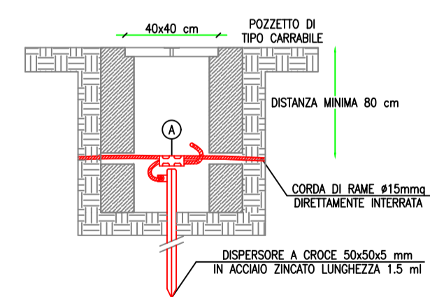
PARTICOLARE POZZETTO DI TERRA (FUORI SCALA)
